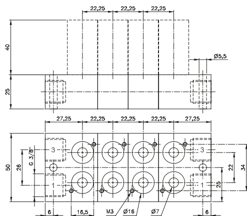
R 3 __ 703 G Furat méret: 15 mm
