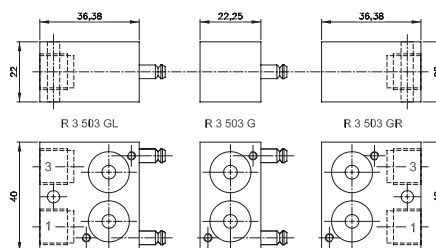
Moduláris alaplap elemei R 3 __ 503 G
