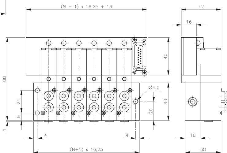
T_16 5__303 343 T típusú szelepekkel felszerelve
