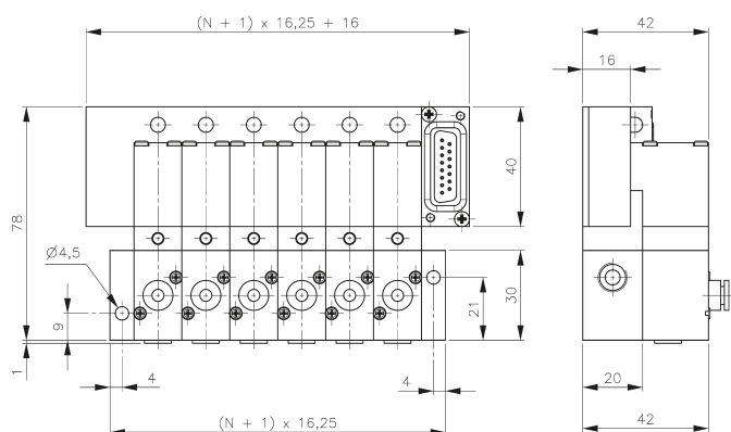
T_16 3__303 343 T típusú szelepekkel felszerelve
