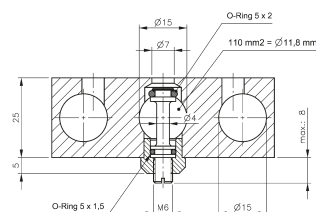
Zárható táplevegő (R 5 703 G D1)
