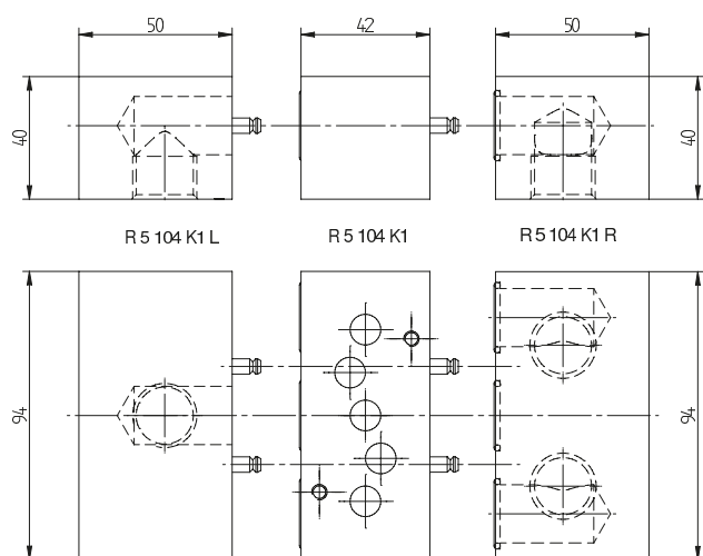
Moduláris alaplap elemei R 5__ 104 K1
