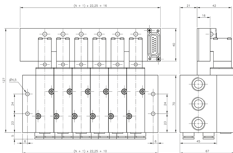
T_22 5_784 704 T típusú szelepekkel felszerelve
