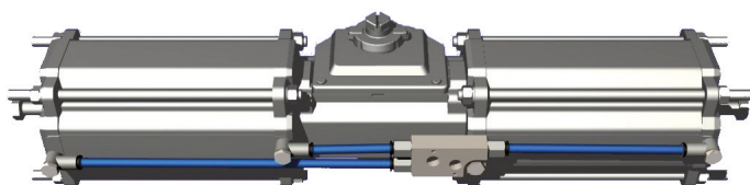
Kettős működésű munkahenger
