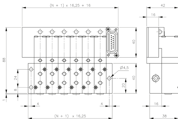
T_16 5__303 303 T típusú szelepekkel felszerelve
