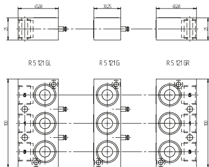
Moduláris alaplapp elemei R 5 __ 121 G
