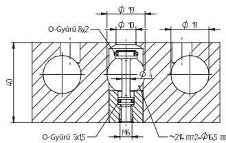
Közbenső elem zárható 1-es csatlakozással (R 5 104 K1)
