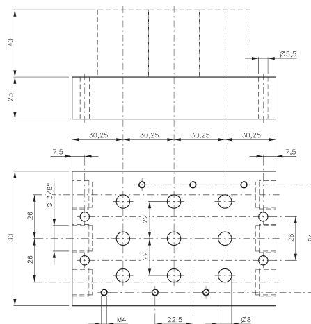
R 5 __ 803 Furat méret: 15 mm
