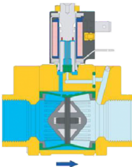
Koaxiális membránszelep
