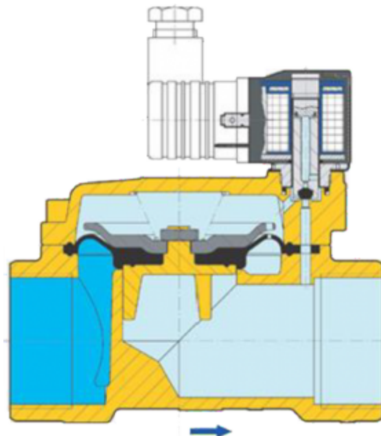
Ülékes membránszelep
